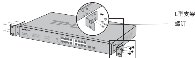
图2-2 L型支架安装示意图
