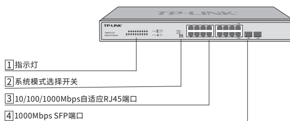
图1-1 前面板示意图
