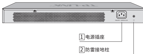
图1-4 后面板示意图
