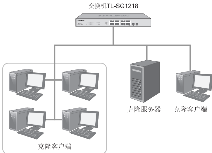
图1-3 网络克隆模式拓扑示例
