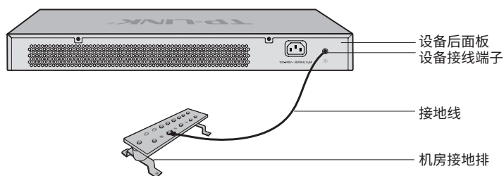
图2-4 接地排连接示意图
